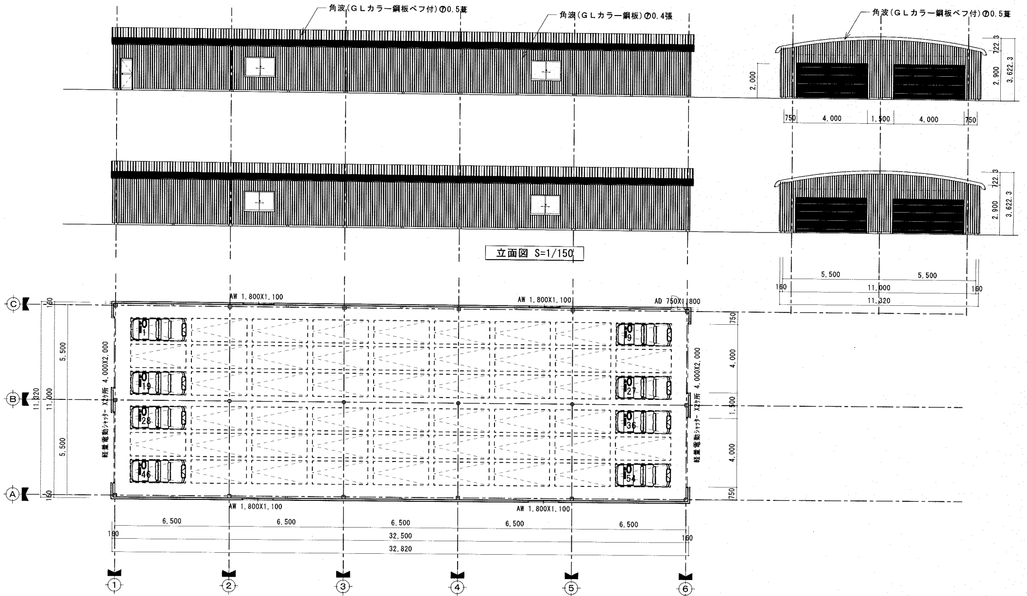
平面図 S=1/150
