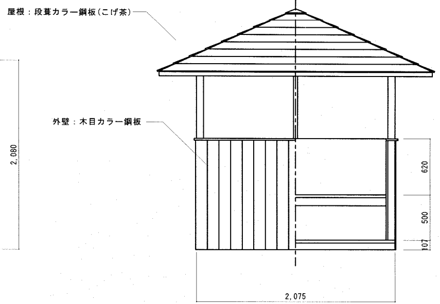
避雷小屋 ライガード M-2020B型
